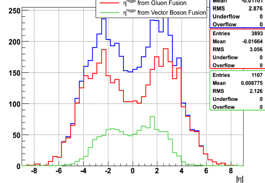
|\eta^{\text{higgs}}| (HZZ4e_150_5k)
